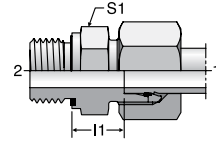
DIN 3852-2 Form E
